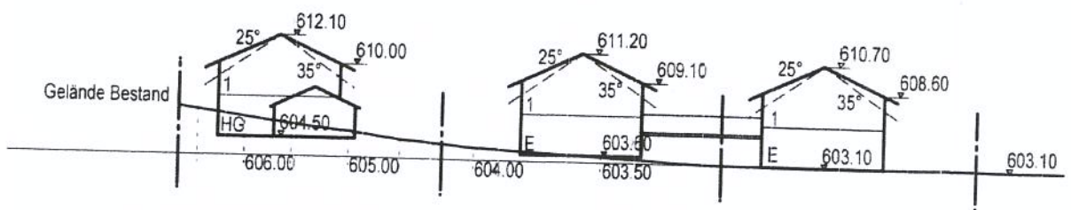
Schema Ansicht Norden
